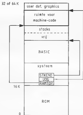
Afb. 1-2 Geheugenindeling na wijzigen RAMTOP
